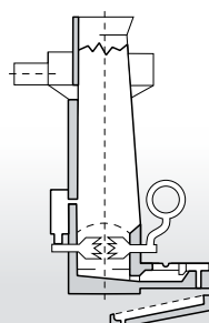
Cupolas \ Cubilote
